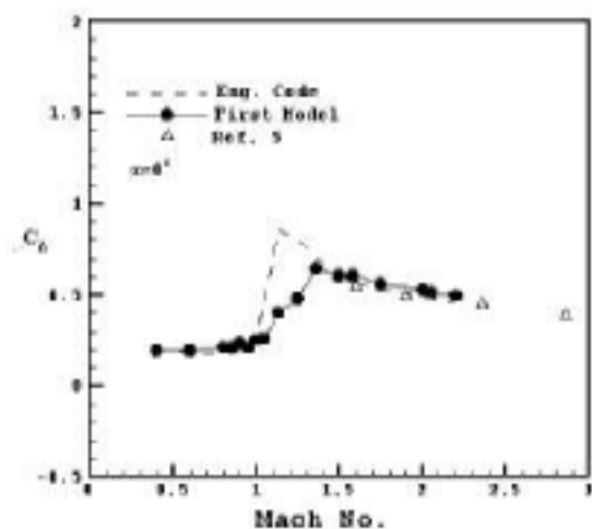
شکل ۷- تغییرات C_d با عدد ماخ در زاویه حمله صفر
