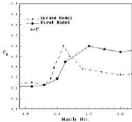
شکل ۸- تغییرات C_d با عدد ماخ در زاویه حمله ۲ درجه برای هر دو مدل
