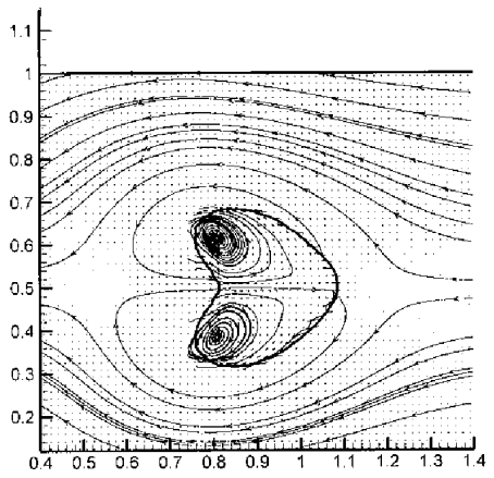
شکل ۱۱ - میدان جریان در داخل و خارج قطره در t=0.3 برای
