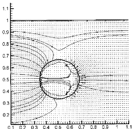
شکل ۷ - میدان جریان در داخل و خارج قطره در t=0.005 برای
