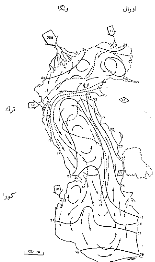
شکل ۳-الف- نمونه‌ای از طرح گردش آب در دریای خزر (بردارهای جریان مسیر حرکت آب را بدون توجه به اندازه سرعت جریان نشان می‌دهند) [۱۶-۱۹].
