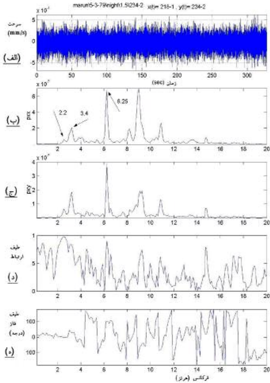
شکل ۴- الف- تاریخچه زمانی سرعت ثبت شده در نقطه‌ای از تاج سد خاکی مارون (واقع در ۱/۴ طولی سمت راست) در آزمایش ارتعاش محیطی ب- چگالی طیف توان رکورد ج- دامنه طیف توان مقاطع رکورد مذکور نسبت به نقطه مرجع واقع در مرکز تاج د- طیف ارتباط دو رکورد مذکور ه- فاز طیف توان مقاطع دو رکورد
