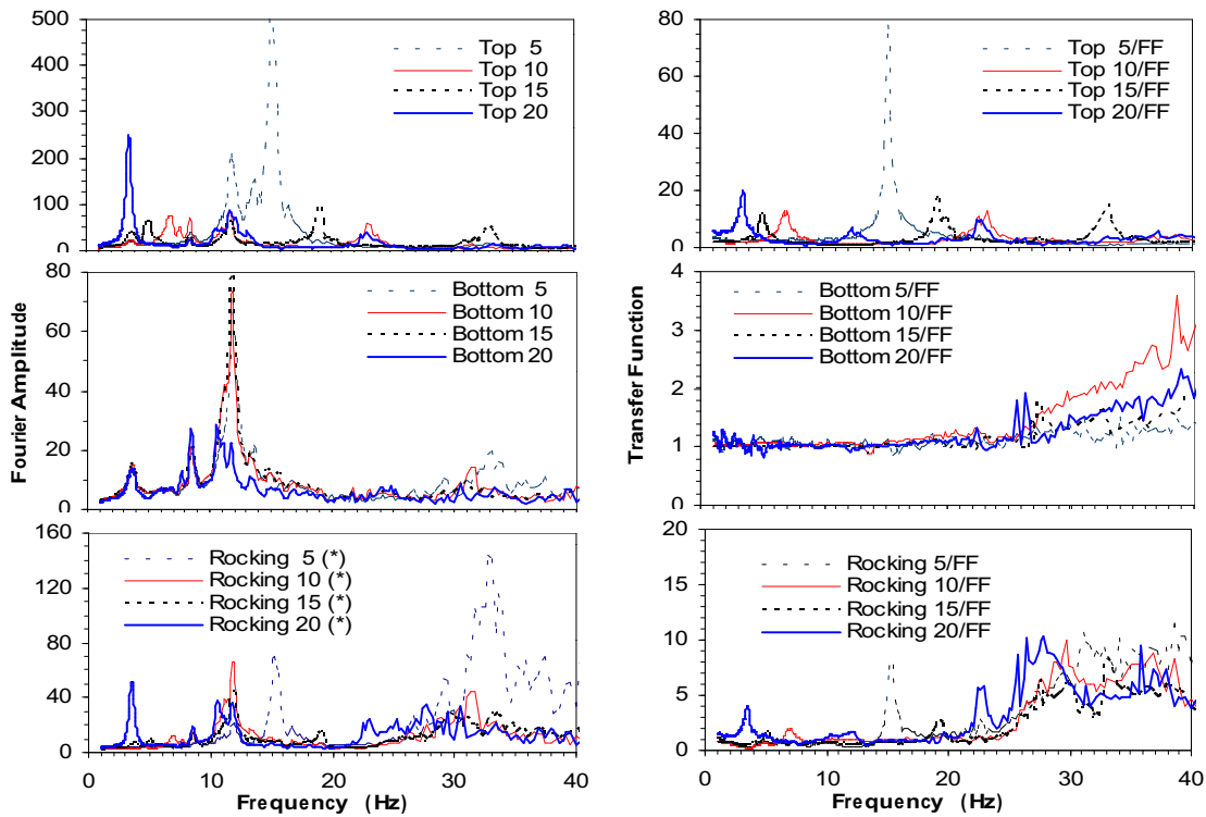
شکل ۱۹- تبدیل فوریه و تابع انتقال پاسخ شتاب نوک مدل‌های سازه‌ای و مدهای افقی و گهواره‌ای پی‌ها نسبت به سطح آزاد تحت زلزله السنترو
