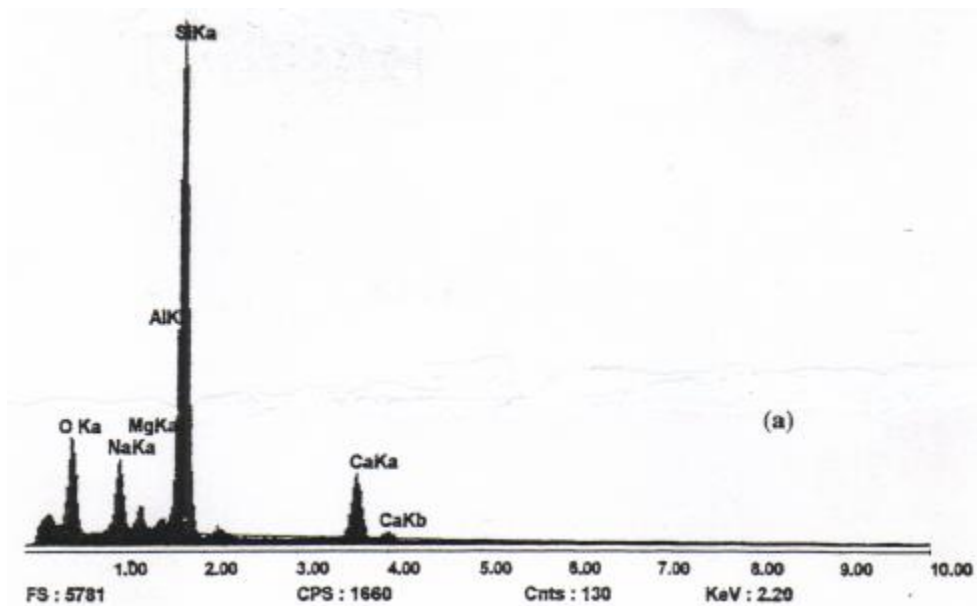
شکل ۷ - آنالیز عنصری EDAX از سطح لایه‌های پوششی \text{SiO}_2 به روش Sol-Gel
