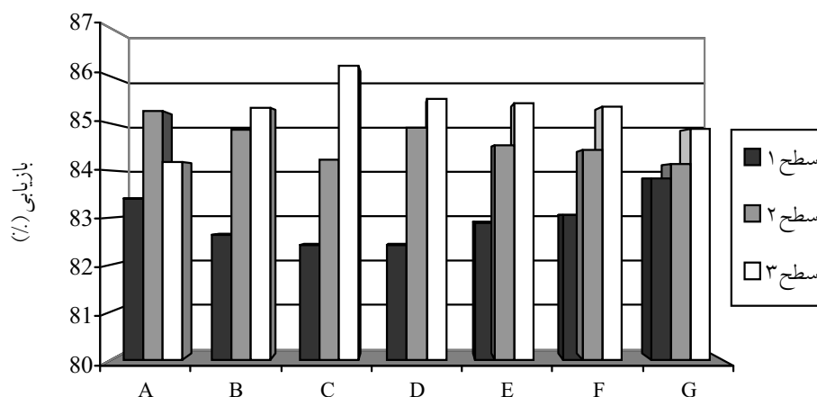
شکل ۱- تأثیر سطوح هفت عامل در بازیابی سنگ معدن کالکوسیتی
