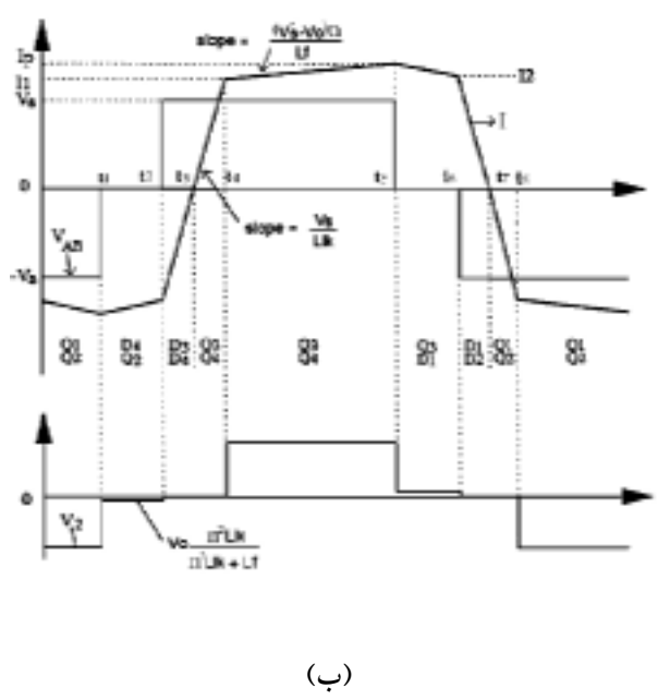
ب- شکل موجهای آن (روشهای A و B)
