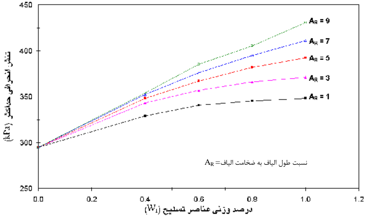
شکل ۷- تغییرات تنش انحرافی حداکثر بر حسب درصد وزنی عناصر تسلیح W_f و نسبت اضلاع عناصر A_R در آزمایش سه‌محوری CD ( s'_c = 100 kPa)
