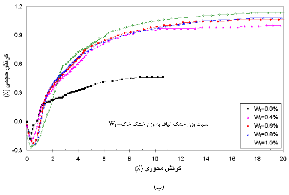
شکل ۶- تغییرات تنش انحرافی (شکل الف) و کرنش حجمی (شکل ب) در آزمایش سه محوری CD ( s'_c=100 kPa ) برای درصدهای وزنی مختلف عناصر تسلیح ( W_f ) و نسبت اضلاع عناصر A_R = 9
