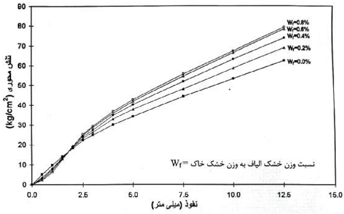
شکل ۱۵- تغییرات تنش محوری بر حسب نفوذ سنبه برای نمونه‌های با نسبت اضلاع عناصر A_R=5 و غرقاب شده به مدت ۲۴ ساعت در آزمایش CBR
