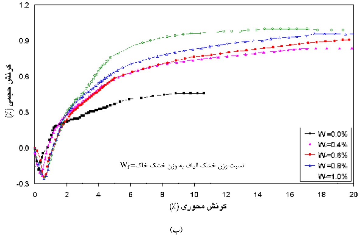
شکل ۴- تغییرات تنش انحرافی (شکل الف) و کرنش حجمی (شکل ب) در آزمایش سه محوری CD ( s'_c = 100 \text{ kPa} ) برای درصدهای وزنی مختلف عناصر تسلیح ( W_f ) و نسبت اضلاع عناصر A_R = 5
