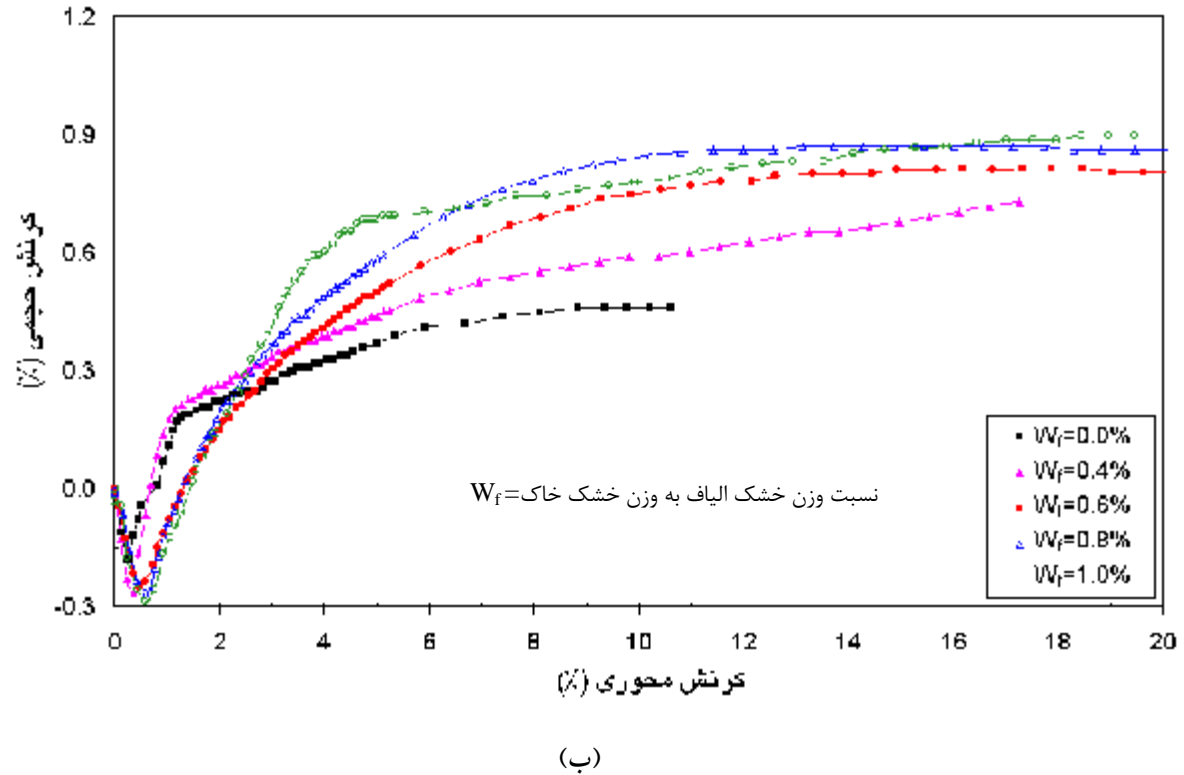
شکل ۳- تغییرات تنش انحرافی (شکل الف) و کرنش حجمی (شکل ب) آزمایش سه محوری CD ( S'_c = 100 \text{ kPa} ) برای درصدهای وزنی مختلف عناصر تسلیح ( W_f ) و نسبت اضلاع عناصر A_R = 3
