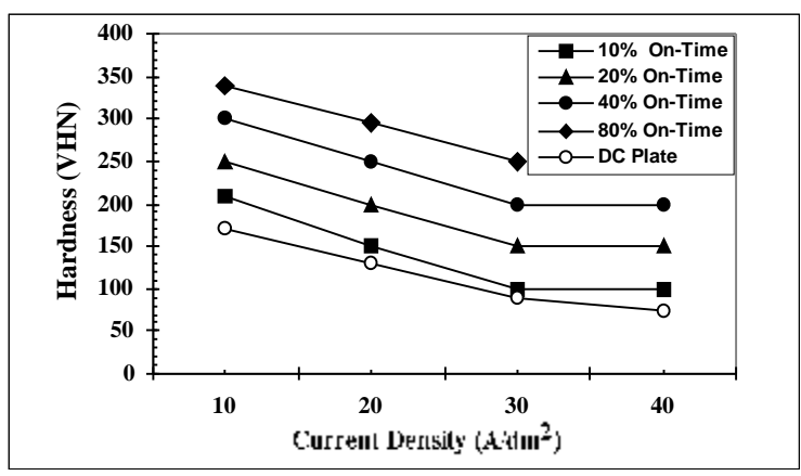
شکل ۶- تاثیر چگالی جریان و درصد زمان روشن در سختی پوشش (فرکانس ۵۰۰ Hz)
