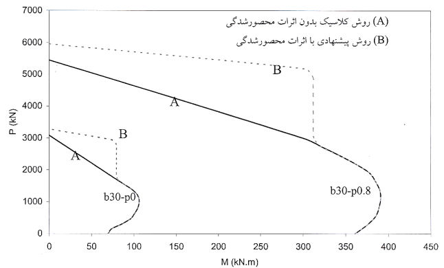
شکل ۷ - نمودار اندرکنش بار محوری - لنگر خمشی نمونه های b30-p0 و b30-p0.8
