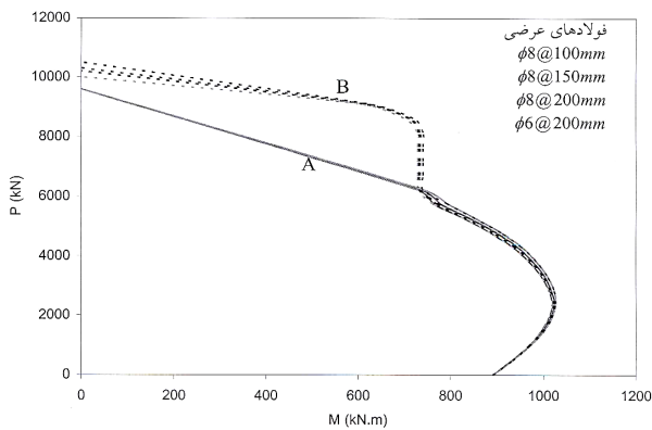
شکل ۹ - نمودار اندرکنش بار محوری - لنگر خمشی نمونه های b45-p0.8 با فولادهای عرضی متفاوت
