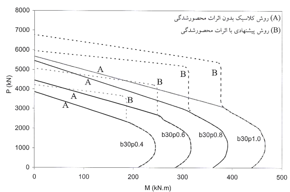
شکل ۱۰ - نمودار اندرکنش بار محوری - لنگر خمشی نمونه های b30-p0.4, b30-p0.6, b30-p0.8, b30-p1.0
