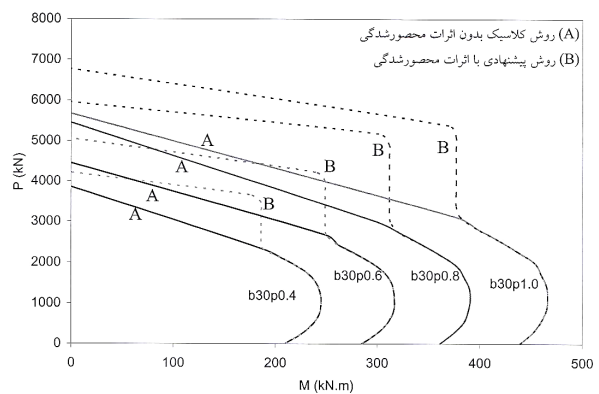
شکل ۱۰ - نمودار اندرکنش بار محوری - لنگر خمشی نمونه های b30-p0.4, p0.6, p0.8, p1.0
