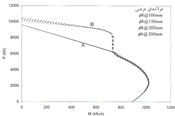
شکل ۹ - نمودار اندرکنش بار محوری - لنگر خمشی نمونه های b30-p0.8 با فولادهای عرضی متفاوت
