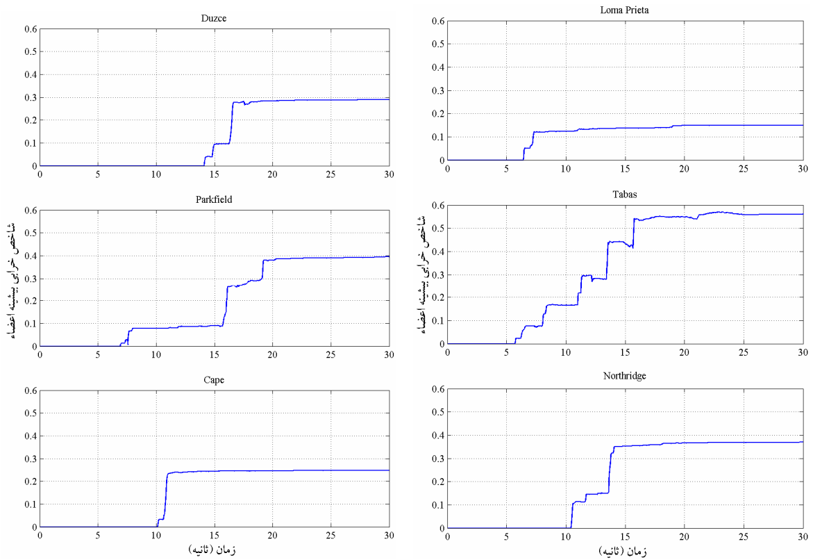
شکل ۱۸- تاریخچه شاخص خرابی بیش از یک عضو برای دوره بازگشت ۲۵۰۰ ساله
