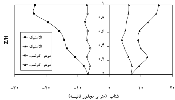
شکل ۳۰- تغییرات شتاب افقی حداکثر در ارتفاع سد ۴۰ متری برای زلزله "ناغان"
