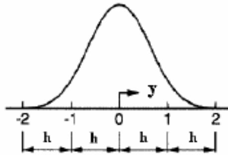
شکل ۴ - تابع اسپلاین محلی \psi_0
