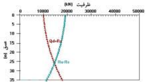
شکل ۶ - ظرفیت باربری و محل صفحه خشی در نرم‌افزار Unipile
