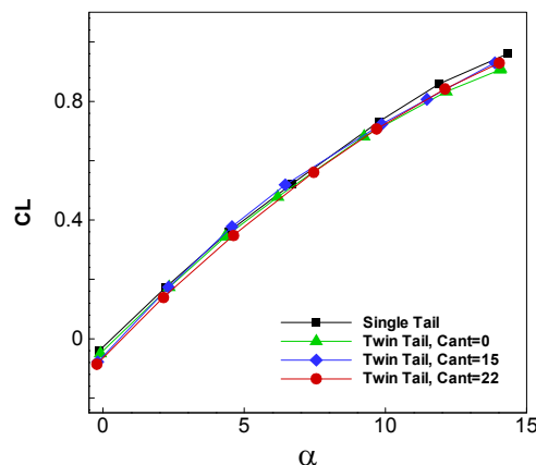
شکل ۶-الف) ضریب برآ در ماخ ۱/۴
