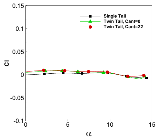
شکل ۷-ج) ضریب گشتاور چرخشی در زاویه جانبی صفر درجه
