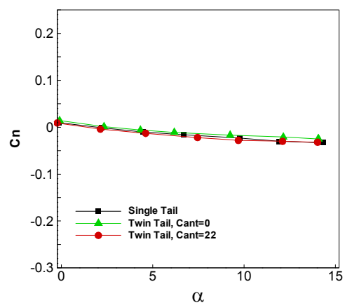
شکل ۷-هـ) ضریب گشتاور جانبی در زاویه جانبی صفر درجه
