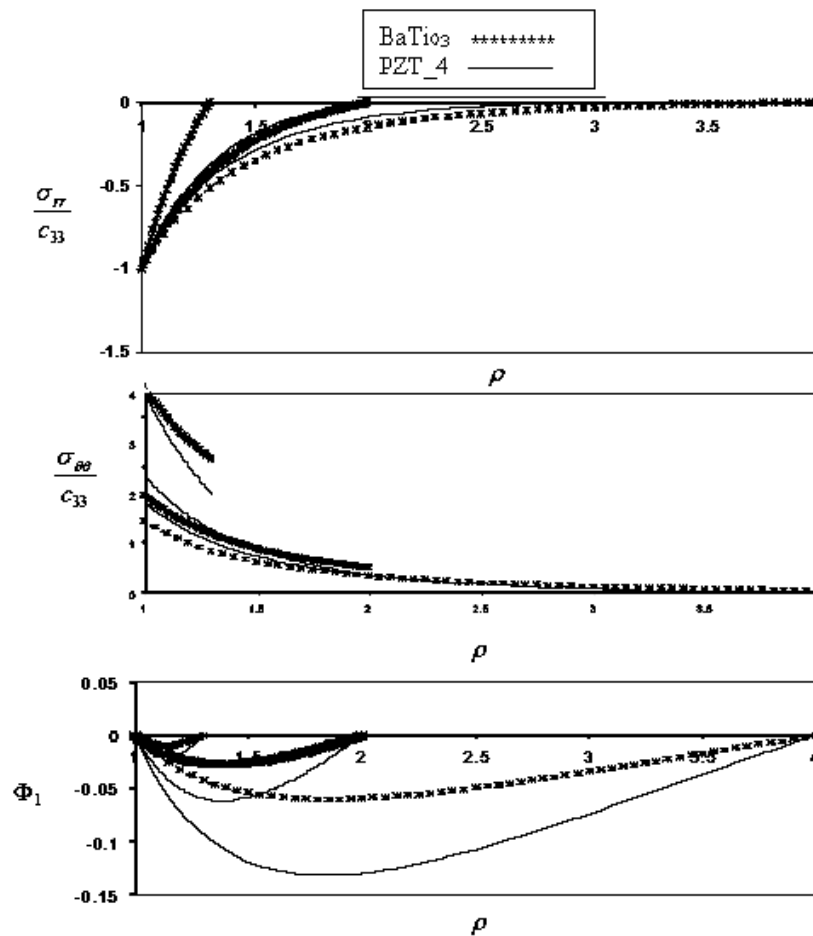
شکل ۲ - حالت اول بارگذاری، اعمال فشار داخلی برای نسبت‌های شعاع \eta = 1.3, 2, 3, 4
