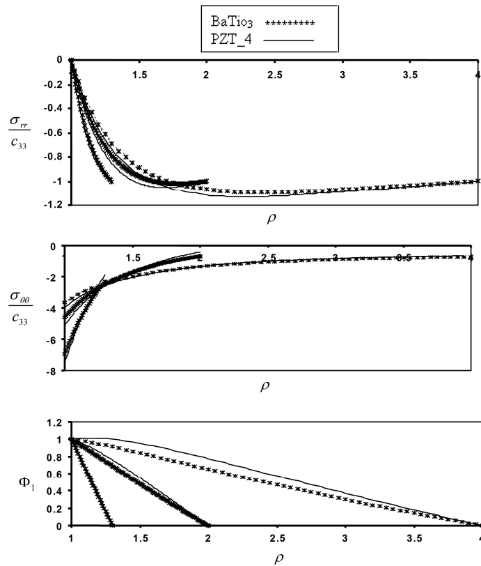
شکل ۷- حالت ششم بارگذاری، اعمال پتانسیل الکتریکی و فشار خارجی برای \eta = 1, 2, 3, 4
