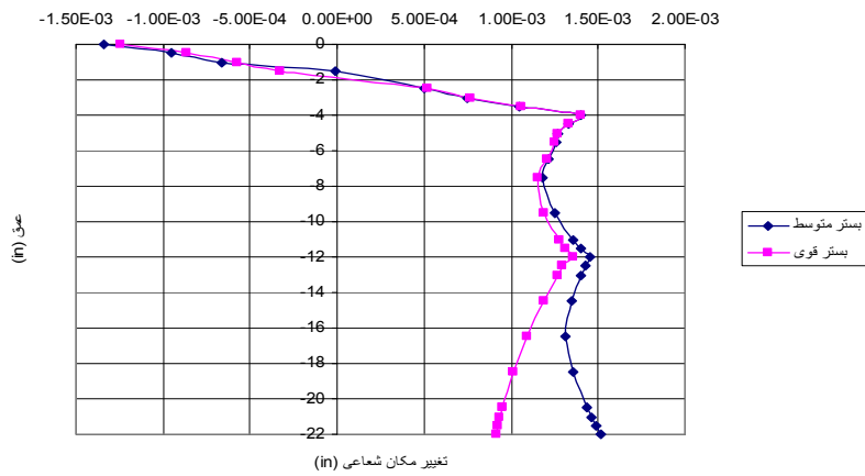
شکل ۴ - مقایسه تغییر مکان شعاعی در دو نوع بستر تحت بار محور ۲۰°، فصل گرم و روسازی نازک
