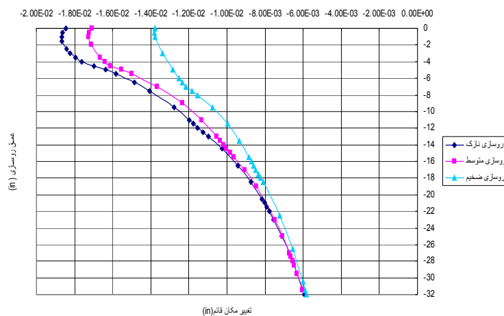
شکل ۶ - مقایسه تغییر مکان قائم در انواع ضخامت روسازیه‌ها تحت بار محور ۲۰ تنی، فصل گرم و بستر قوی
