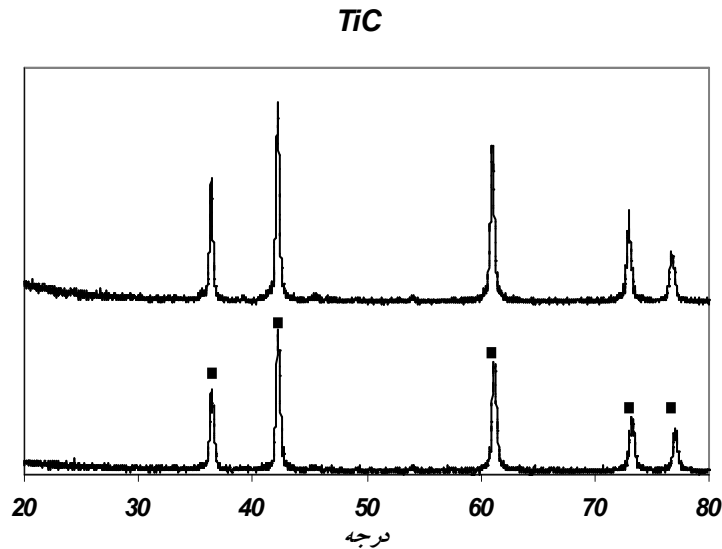
شکل ۵- تحلیل (XRD) باقی مانده آزمایش (TGA) برای نمونه‌های آناتاز- کک که به مدت ۵۰ (پایین) و ۱۰۰ (بالا) ساعت آسیاکاری شده‌اند.
