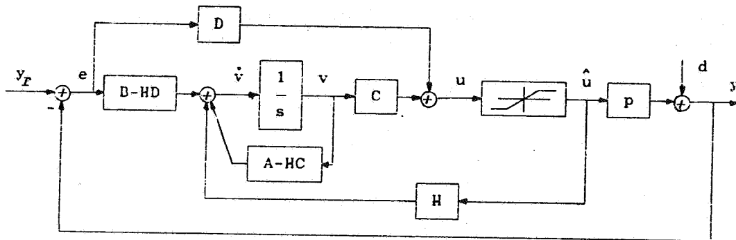
شکل ۱۵- دیاگرام پس‌خور معادل با IMC همراه با آنتی‌واینده
