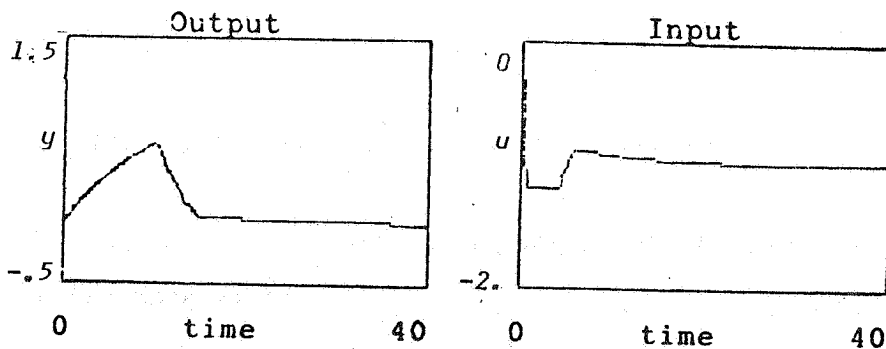
شکل ۱۶- پاسخ نسبت به تغییر d با کنترل کننده پس‌خور معادل IMC ، با وجود محدودیت در ورودی و آنتی‌واینده پیشنهادی کامپیو موری (مثال ۱)
