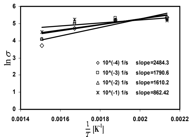
شکل ۱۰- منحنی تغییرات \ln \sigma بر حسب معکوس دما در نرخ کرنشهای مختلف.
