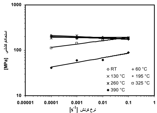
شکل ۲- تغییرات استحکام کششی (UTS) با نرخ کرنش در دماهای مختلف
