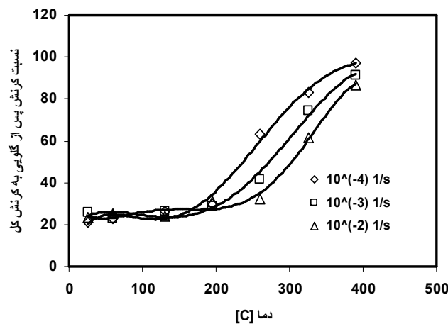
شکل ۹- تغییرات درصد کرنش ناهمگن به کرنش کل بر حسب دما در نرخ کرنشهای مختلف.
