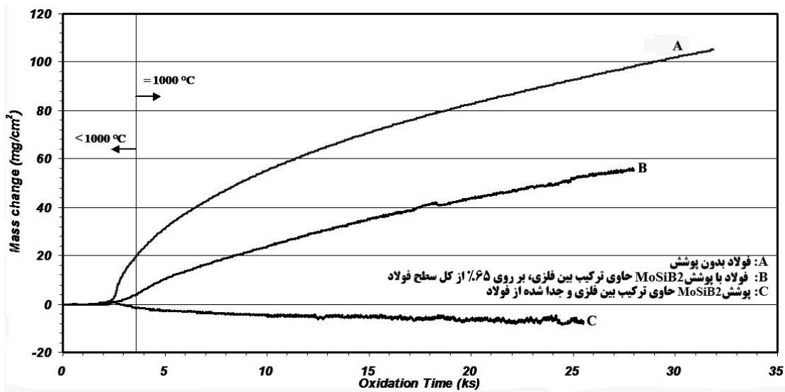
شکل ۶ - نمودارهای اکسایش پیوسته در دمای 1000^\circ\text{C} برای زیرلایه فولادی بدون پوشش و پوشش دار و ترکیب \text{MoSiB}_2 بدون زیرلایه (نسبت سطح پوشش به کل سطح برای نمونه پوشش دار، برابر با ۶۵٪ می باشد).
