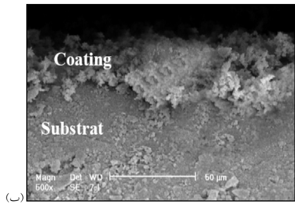
شکل ۵- مورفولوژی سطح (الف) و مقطع عرضی (ب) پوششهای کامپوزیتی HA-3YSZ
