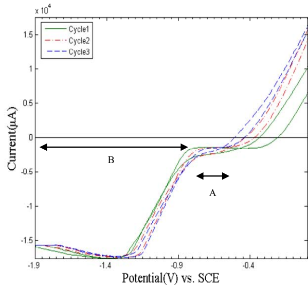
شکل ۱- نمودار CV الکترولیت بر پایه کبالت بر زیر لایه طلا با آهنگ روبش 15 \text{ mVs}^{-1} .
