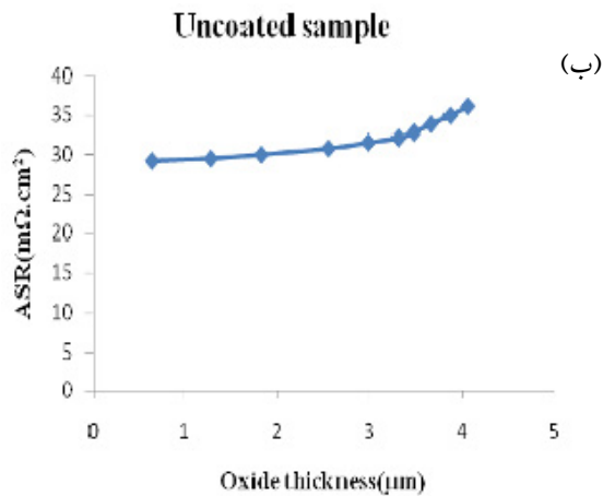
شکل ۳- ASR به عنوان تابعی از ضخامت لایه اکسیدی در اکسیداسیون همدا برای نمونه‌های (الف) پوشش دار و (ب) بدون پوشش.
