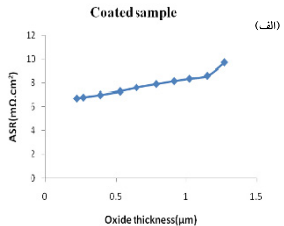
شکل ۳- ASR به عنوان تابعی از ضخامت لایه اکسیدی در اکسیداسیون همدا برای نمونه‌های (الف) پوشش دار و (ب) بدون پوشش.
