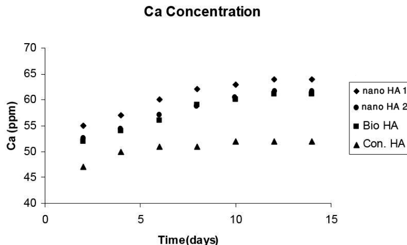
شکل ۶- نمودار تغییرات غلظت یون کلسیم محلول شبیه‌سازی شده بدن حاوی هیدروکسی آپاتیت نانوساختار تهیه شده به روش سل-ژل (nano HA1)، هیدروکسی آپاتیت نانوساختار تهیه شده به روش فعالسازی مکانیکی (nano HA2)، آپاتیت بیولوژیکی (Bio HA) و هیدروکسی آپاتیت تجارتي (Con. HA).
