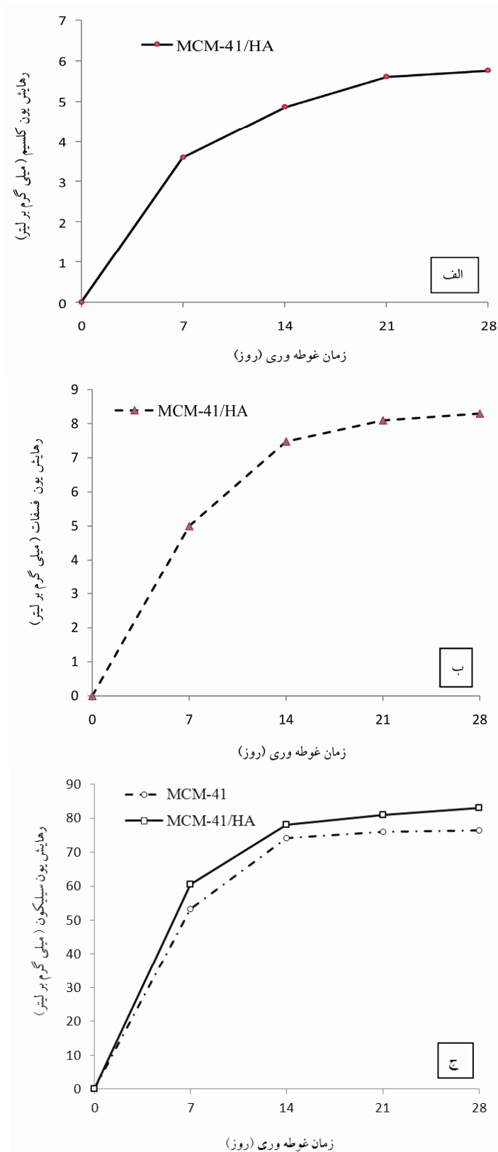
شکل ۴- مقدار رهائش یون الف) کلسیم در نمونه MCM-41/HA، ب) فسفر نمونه MCM-41/HA و ج) سیلیکون در نمونه MCM-41 و MCM-41/HA در آب دیونیزه شده در دمای ۳۷°C.
