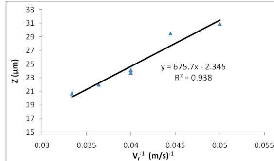
شکل ۴- ارتباط ضخامت فویل ریخته ریزی شده آلیاژ یونیتیکا با سرعت خطی دیسک مبرد در شرایط فشار تزریق مذاب، فاصله نازل تا دیسک و دمای مذاب ثابت.
