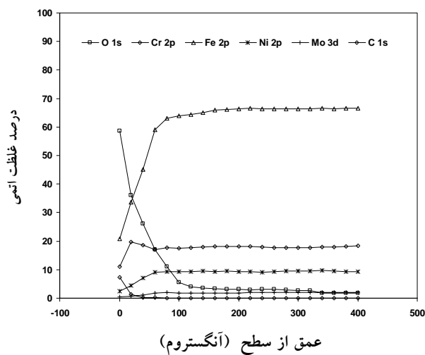
شکل ۷- پروفیل غلظتی عناصر از سطح به عمق فولاد زنگ‌نزن ۳۱۶ کم کربن در پتانسیل ۰/۵ ولت.
