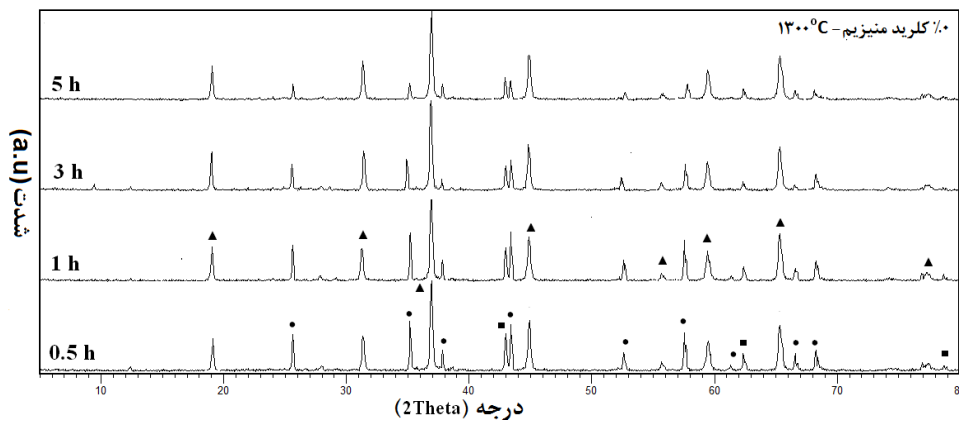
شکل ۱- نتایج تحلیل فازی ترکیبات بدون افزودنی کلرید منیزیم پخته شده در دمای 1300^{\circ}\text{C} و در زمان‌های مختلف ■: Periclase, ▲: Spinel, ●: Corundum
