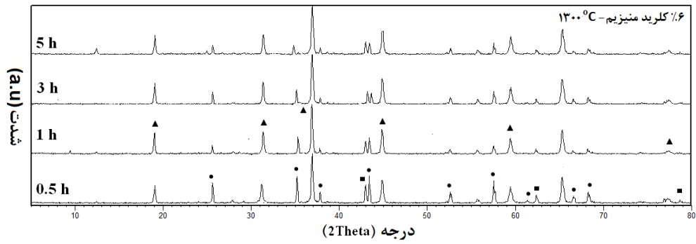
شکل ۲- نتایج تحلیل فازی ترکیبات حاوی ۶ درصد کلرید منیزیم پخته شده در دمای 1300^{\circ}\text{C} و در زمان‌های مختلف
