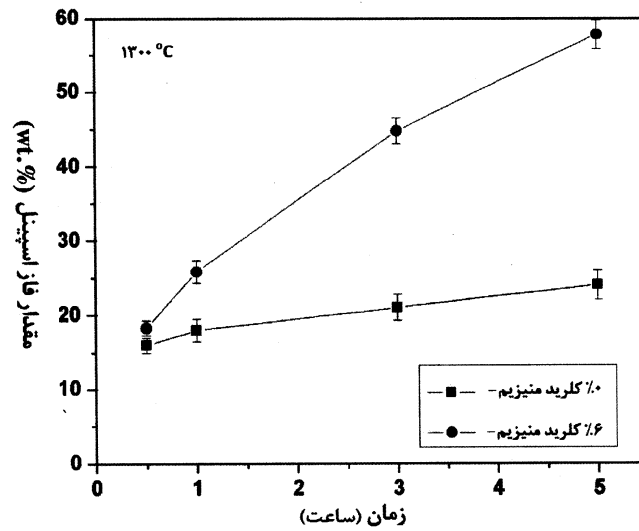
شکل ۳- تاثیر زمان پخت بر مقدار اسپینل تشکیل شده در ترکیبات بدون افزودنی و حاوی ۶ درصد کلرید منیزیم پخته شده در دمای 1300^{\circ}\text{C}
