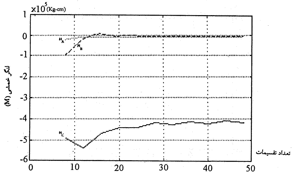
شکل (۴-الف) - مقایسه لغر خمشی نقاط A، B و C محافظ تونل شکل ۳ برای تعداد متفاوت المانها
