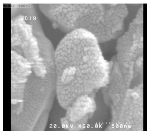
شکل ۳- تصویر میکروسکوپ الکترونی روبشی از شکل و اندازه ذرات سرامیک‌ها
