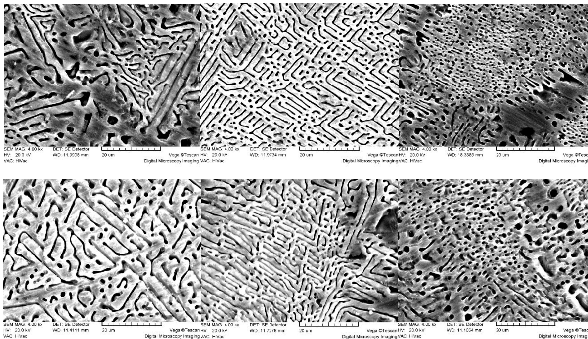
شکل ۷- ریزساختار SEM از مقاطع شعاعی استوانه ریختگی یوتکتیک \text{Al-13.8\%Mg}_2\text{Si} پس از ریخته‌گری گریز از مرکز (تصاویر بالا مربوط به نمونه فاقد جوانه‌زا و تصاویر پایین مربوط به نمونه حاوی یک درصد وزنی ماده جوانه‌زای \text{Al-5Ti-B} هستند)
