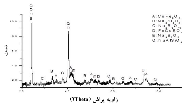
شکل ۵- الگوی XRD نمونه عملیات حرارتی شده در دمای 521^\circ\text{C} درجه سانتی گراد
