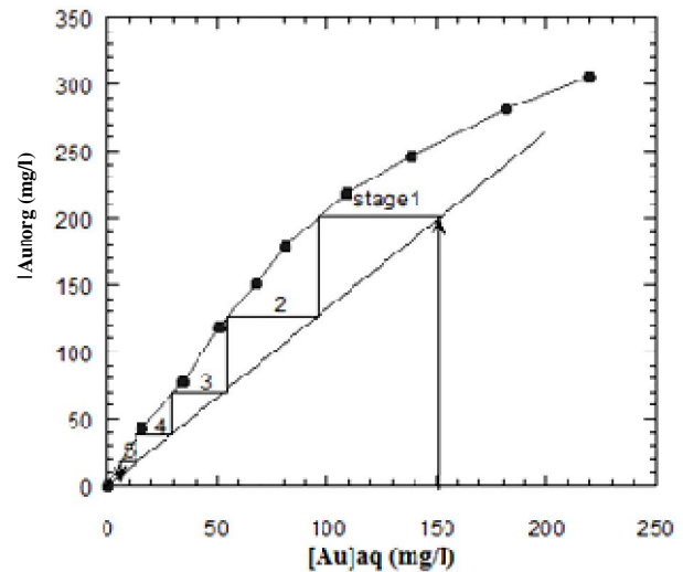
شکل ۳- نمودار هم‌دم و مک‌کیب-تیلی استخراج طلا توسط ۰.۴۰ (v/v)٪ حجمی اوکتانول از ۳ مول بر لیتر اسید کلریدریک
