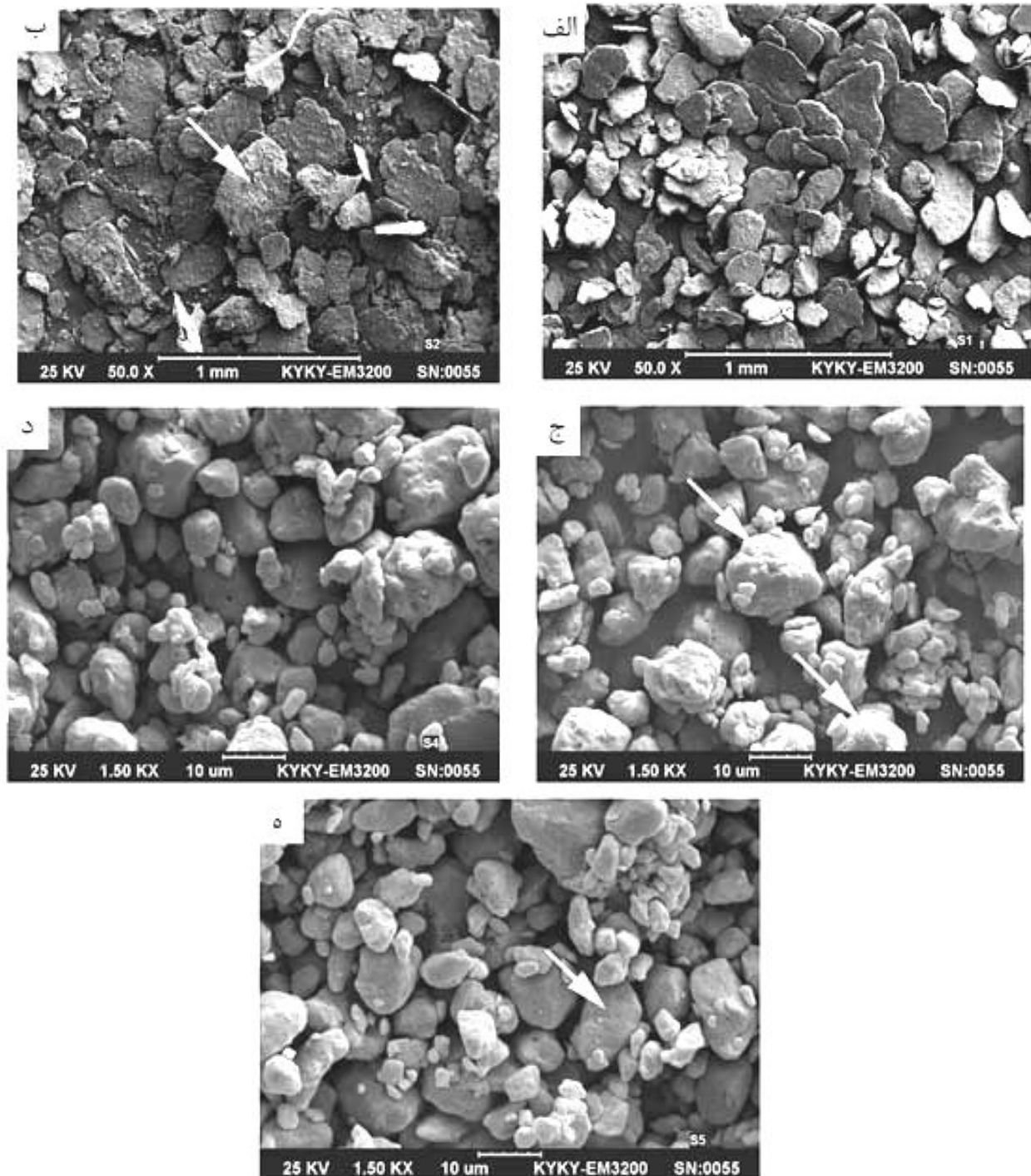
شکل ۱- تصاویر میکروسکوپ الکترونی روبشی از تغییر ریخت مخلوط پودری در زمان‌های مختلف آسیاب:
