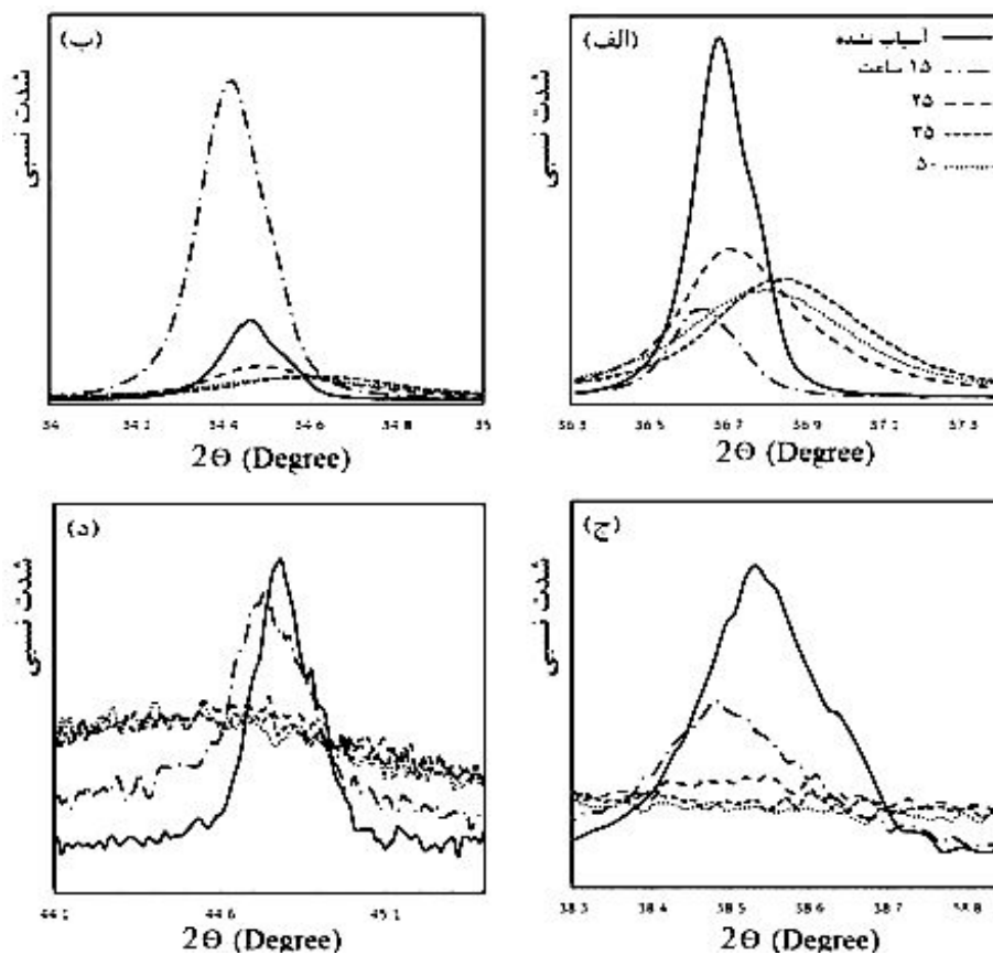
شکل ۴- الگوهای XRD مخلوط پودری در زمان‌های مختلف آسیاب مربوط به قله‌های:
