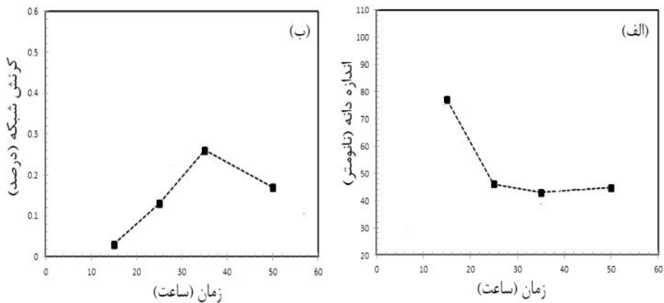
شکل ۵- تغییرات (الف) اندازه دانه و (ب) گرنش شبکه بر حسب زمان آلیاژسازی مکانیکی
