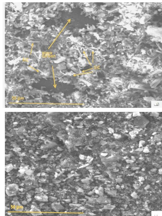
شکل ۹. تصویر میکروسکوپی الکترونی روبشی مقطع شکست برای نمونه‌های الف) K5.5 و ب) K3.5
