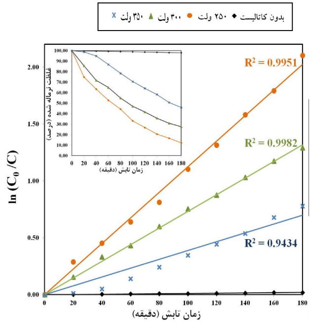
شکل ۳- تغییرات \ln(C_0/C) با زمان تابش امواج فرابنفش برای لایه‌های کامپوزیتی رشد داده شده در مدت زمان ۵ دقیقه، تحت ولتاژهای مختلف در الکترولیت با غلظت ۱۰ گرم در لیتر فسفات سدیم و ۵ گرم در لیتر اکسید نیکل
