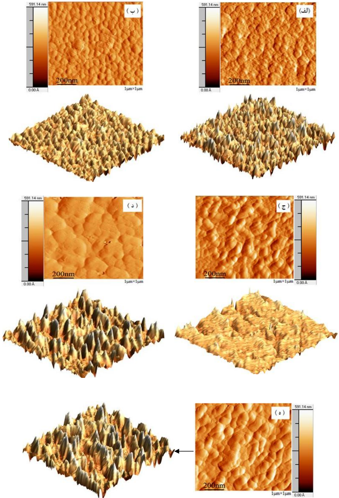
شکل ۴- تصاویر میکروسکوپی روبشی لایه‌های نازک نئودیمیوم آهن بور در دمای آنیل مختلف: الف) ۴۵°، ب) ۵۰°، ج) ۵۵°، د) ۶۰° و ه) ۶۵° درجه سانتی‌گراد
