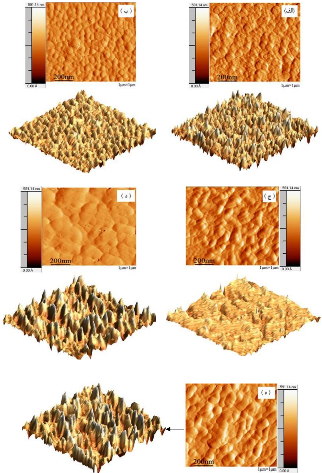
شکل ۴- تصاویر میکروسکوپی روبشی لایه‌های نازک نئودیمیوم آهن بور در دمای آنیل مختلف:
