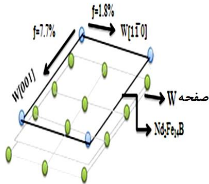
شکل ۱- ارتباط بلورشناسی شبکه بین لایه تنگستن و فاز مغناطیسی نئودیمیوم آهن بور
