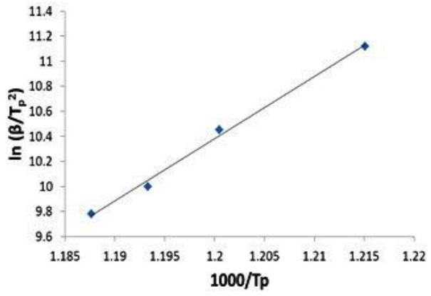
شکل ۲۰- نمودار آرنیوس مربوط به استحاله شیشه‌ای شدن در آلیاژ Fe 55 Cr 18 Mo 7 B 16 C 4
