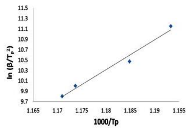
شکل ۱۹- نمودار آرنیوس مربوط به استحاله شیشه‌ای شدن در آلیاژ Fe 52 Cr 18 Mo 7 B 16 C 4 Nb 3
