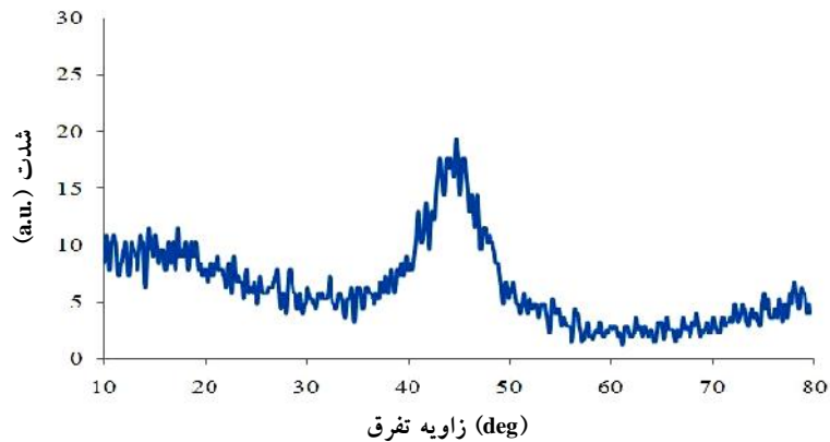
شکل ۷- منحنی تفرق اشعه ایکس آلیاژ \text{Fe}_{55}\text{Cr}_{18}\text{Mo}_7\text{B}_{16}\text{C}_4 در حالت آمورف
