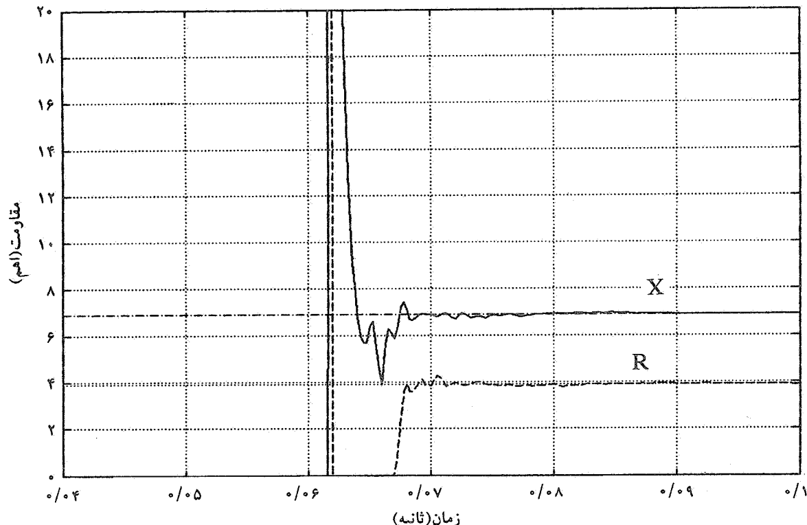
شکل ۲ - راکتانس و مقاومت اندازه گیری شده با استفاده از الگوریتم تعقیب نوع خط: فاز a به زمین طول خط: ۲۰۰ کیلومتر محل خط: ۱۰۰ کیلومتر از رله زاویه وقوع خطاری موج ولتاژ فاز a: ۹۰ درجه
