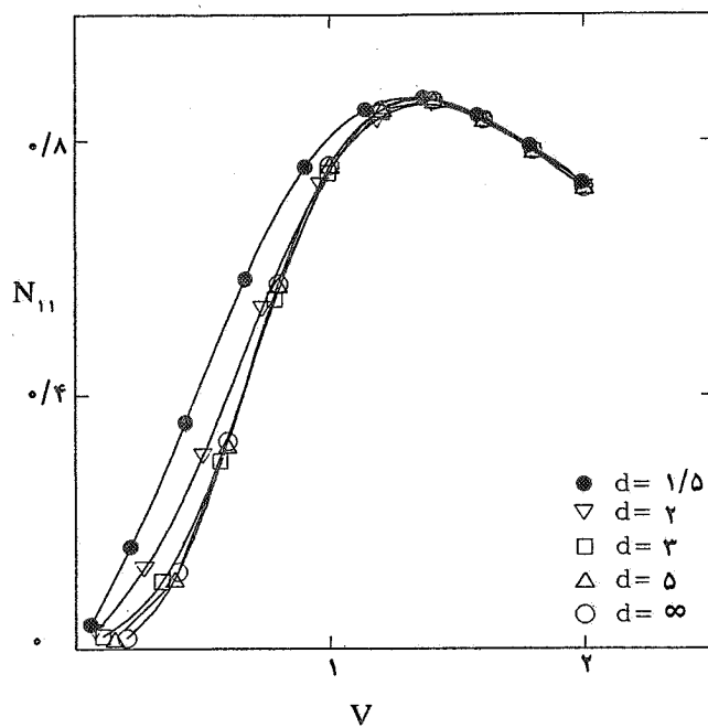
شکل ۱۶ - ضریب میرایی حرکت افقی کره
