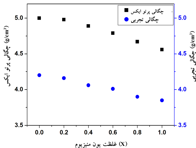
شکل ۵- نمودار تغییرات چگالی تجربی و چگالی پرتو ایکس با جانشانی منیزیم در فریت
