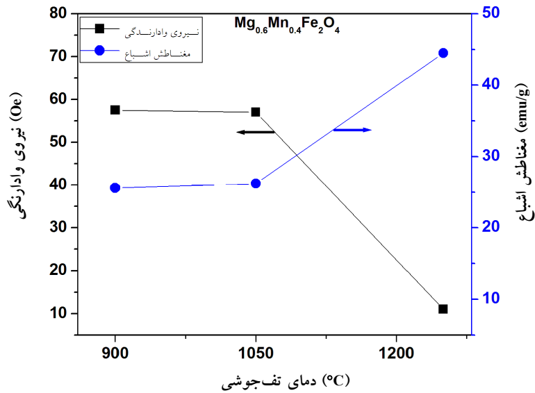
شکل ۱۳- روند تغییرات نیروی وادارندگی و مغناطش اشباع برای نمونه x = 0.6 در سه دمای تفجوشی ۹۰۰، ۱۰۵۰ و ۱۲۵۰ درجه سانتی گراد
