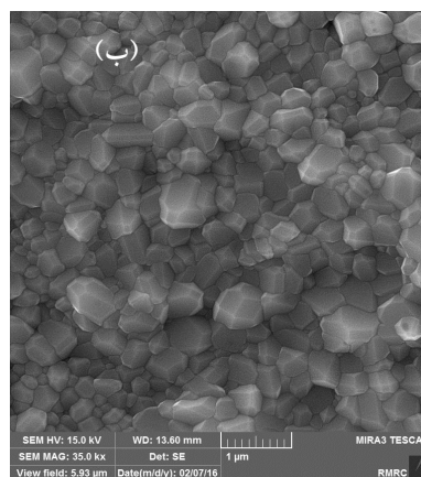
شکل ۹- تصاویر میکروسکوپی الکترونی روبشی نشر میدانی از سطح مقطع شکست: الف) نمونه خام حاصل از ریخته‌گری دوغابی، ب) نمونه شکل‌دهی شده به‌روش ریخته‌گری دوغابی و سپس تف‌جوشی شده به‌روش پلاسما جرقه‌ای، ج) نمونه پودری تف‌جوشی شده به‌روش پلاسما جرقه‌ای
