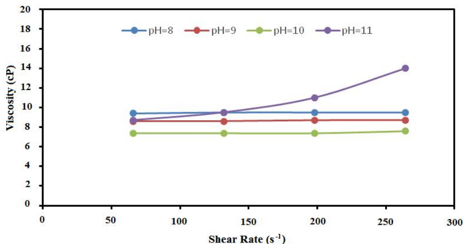
شکل ۳- نمودار گرانروی- نرخ برشی دوغاب پودر نانوکامپوزیتی آلومینا/ ایتریا به عنوان تابعی از اسیدیته
