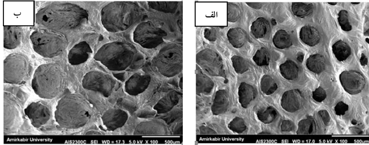
شکل ۳- ساختار میکروسکوپی داربست همگن: الف) نوع ۱ و ب) نوع ۲
