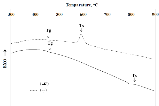
شکل ۳- نمودارهای آنالیز حرارتی مربوط به شیشه‌های 5^\circ\text{GeO}_2-(5^\circ-x)\text{PbO}-x\text{CaO} در حضور:
