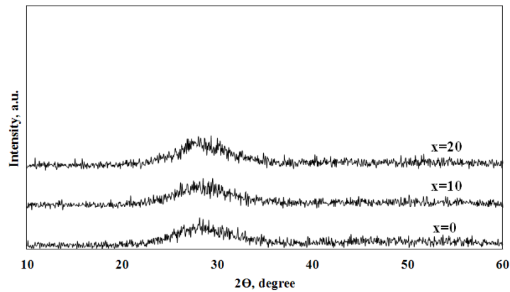
شکل ۲- الگوهای پراش پرتو ایکس مربوط به شیشه‌های 5^\circ\text{GeO}_2-(5^\circ-x)\text{PbO}-x\text{SrO} در حضور صفر، ۱۰ و ۲۰ درصد مولی اکسید کلسیم
