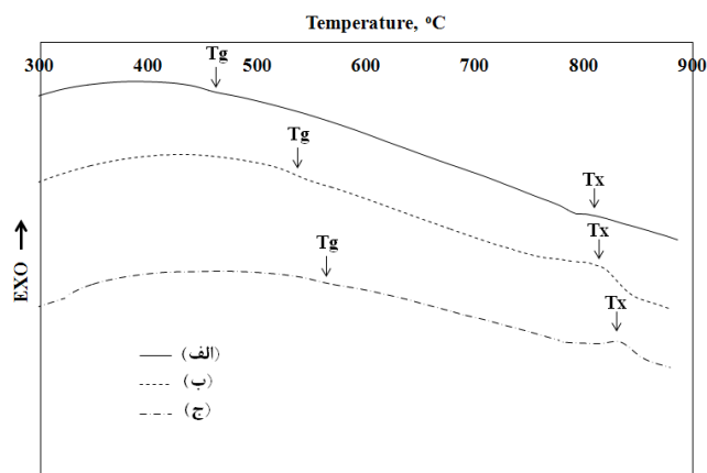
شکل ۴- نمودارهای آنالیز حرارتی مربوط به شیشه‌های 5^\circ\text{GeO}_2-(5^\circ-x)\text{PbO}-x\text{SrO} در حضور:
