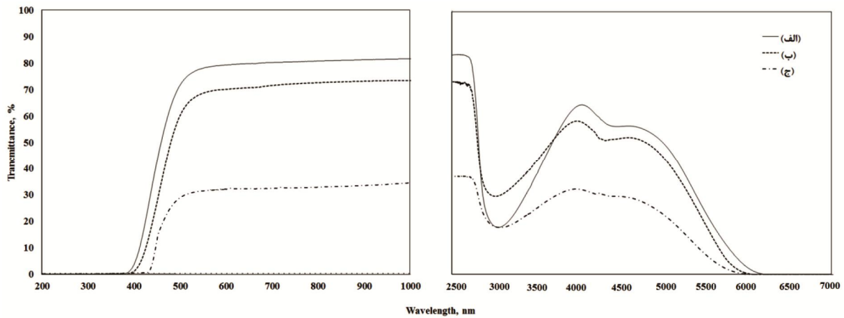
شکل ۶- نمودارهای عبورپذیری مربوط به شیشه‌های 50\text{GeO}_2-(50-x)\text{PbO}-x\text{CaO} در حضور: (الف) صفر، (ب) 10^\circ و (ج) 20^\circ درصد مولی اکسید کلسیم (با ضخامت سه میلی‌متر)
